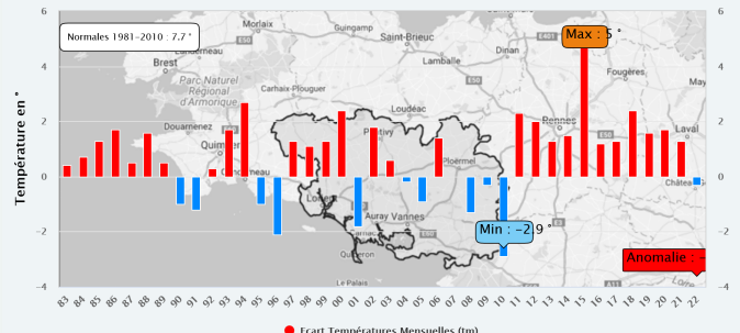
Morbihan – Anomalies Températures Mensuelles (tm) Decembre (1983–2022) A.M.B. le 12/01/2023
