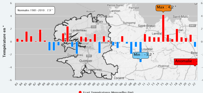
Finistère – Anomalies Températures Mensuelles (tm) Decembre (1983–2022) A.M.B. le 12/01/2023
