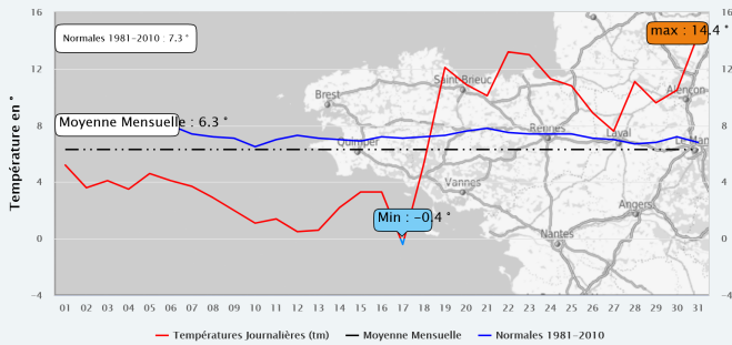
Bretagne – Températures Journalières (tm) Decembre 2022 Association Météo-Bretagne le 12/01/2023
