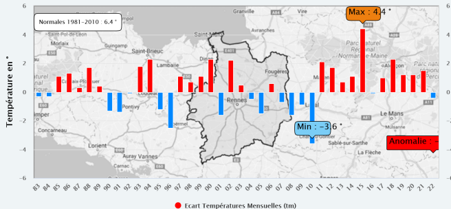
Ille et Vilaine – Anomalies Températures Mensuelles (tm) Decembre (1983–2022) A.M.B. le 12/01/2023
