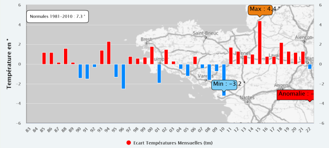
Bretagne – Anomalies Températures Mensuelles (tm) Decembre (1983–2022) A.M.B. le 12/01/2023
