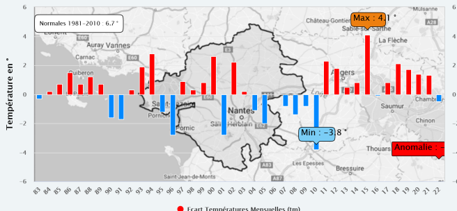
Loire Atlantique – Anomalies Températures Mensuelles (tm) Decembre (1983–2022) A.M.B. le 12/01/2023
