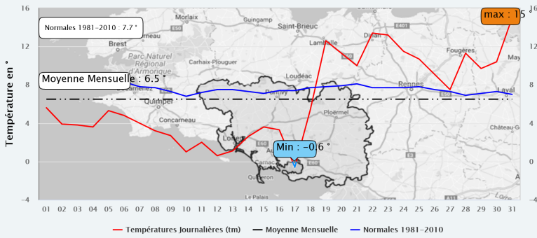
Moyenne journalière des 17 stations du réseau MBdata (Saint-Malo-des-trois-fontaines / Quiberon / Mauron / Cléguer - Sénébret / Pontivy / Meslan - La Grande Métairie / Surzur / Evellys / Ile Arz Keriane) http://cb.asso-mb.fr/Journal_MB/MB/Temp_Mensuelle_Moy1_56_tm_12.png
