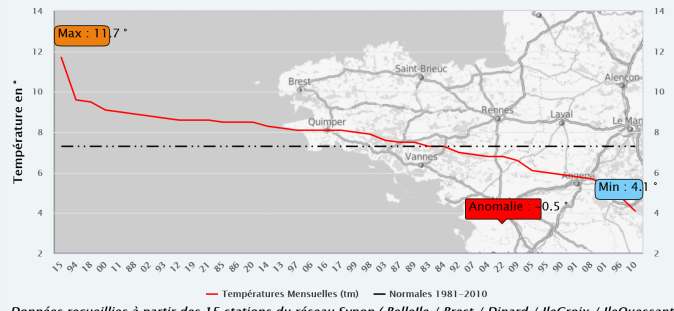
Bretagne – Températures Mensuelles (tm) Decembre (1983-2022) Association Météo-Bretagne le 12/01/2023
