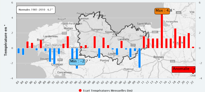
Cotes d Armor – Anomalies Températures Mensuelles (tm) Decembre (1983–2022) A.M.B. le 12/01/2023
