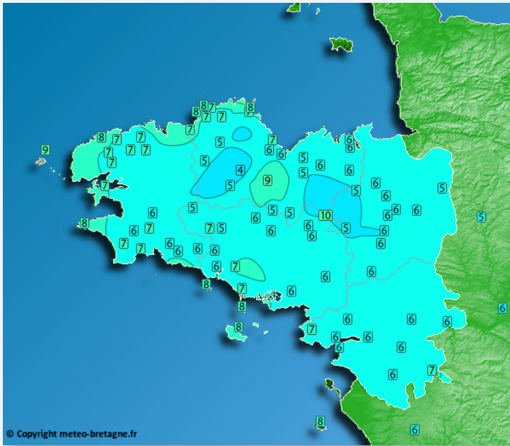
Bretagne – Températures Journalières (tm) Decembre 2022 Association Météo-Bretagne le 12/01/2023
